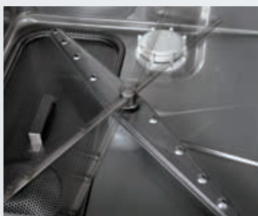
Brazos separados de lavado y aclarado
